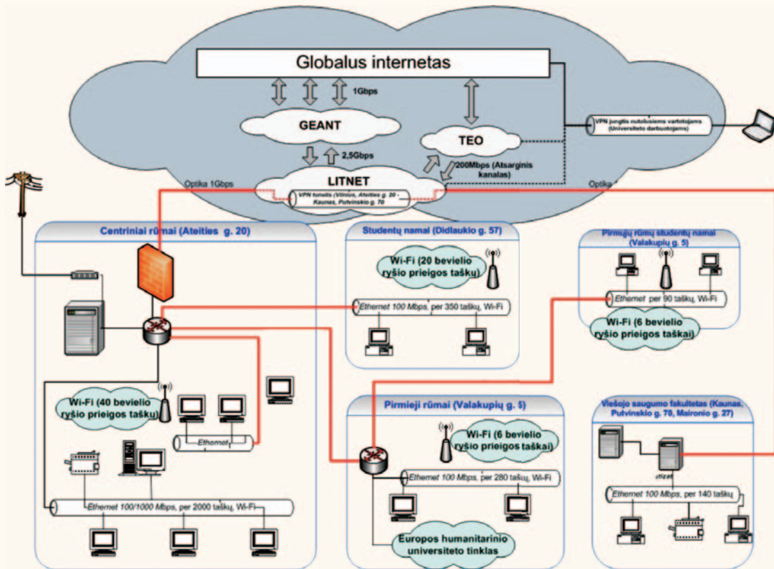
Universiteto kompiuterių tinklo struktūrinė schema ir ryšiai su kitais tinklais
